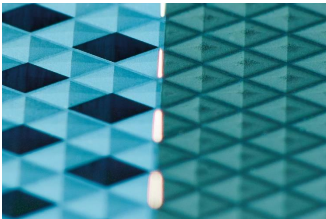
Bild 1: Der sequentielle Einsatz des UKP-Lasers zum Reinigen und Polieren des Bauteils nach der Strukturerzeugung reduziert die Nacharbeiten und sorgt für gezielte Poliereffekte. © Fraunhofer ILT, Aachen / Volker Lannert.
