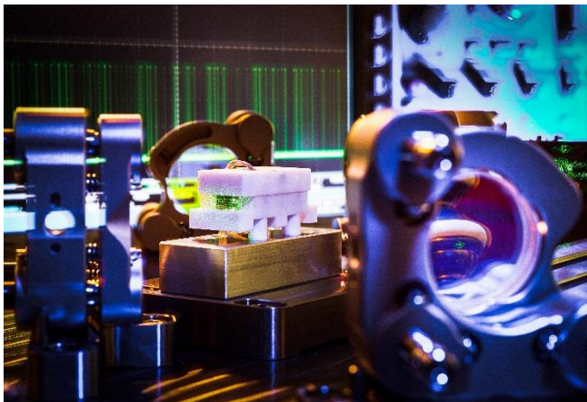
Bild 1: Parametrische Quelle für verschränkte Photonen. © Fraunhofer ILT, Aachen / Volker Lannert.
