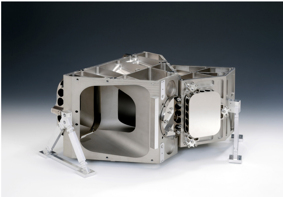
Blick in ein Leichtgewichtsgehäuse einer Metalloptik. © Fraunhofer IOF/Michael Weimer
